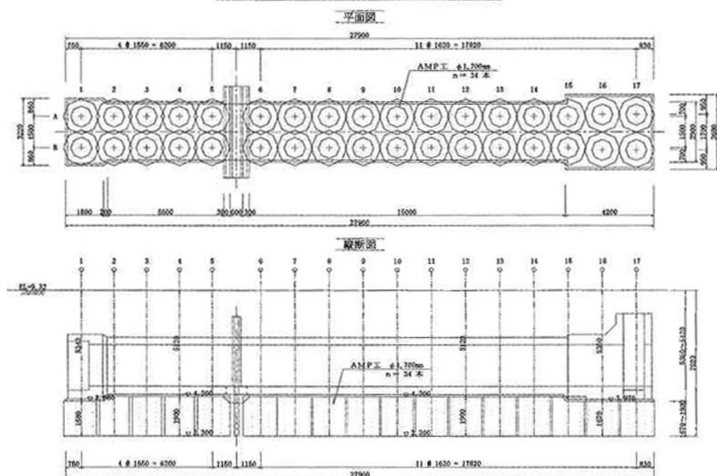
地盤改良工 施工範囲詳細図 S=1/100
