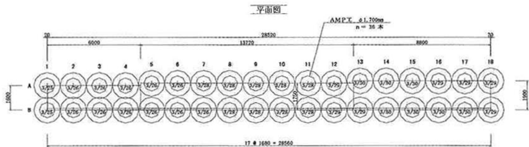
地盤改良工 施工範囲詳細図 S=1/100
